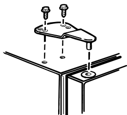
Installation de la charnière à gauche
